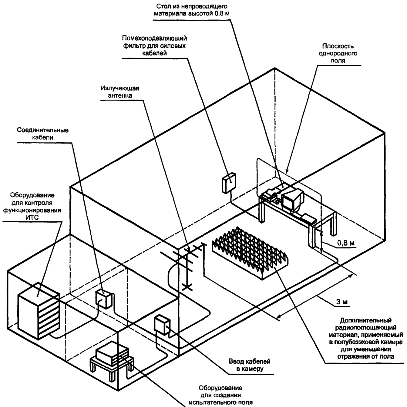
Рисунок 2 — Пример средств испытаний, удовлетворяющих требованиям стандарта
