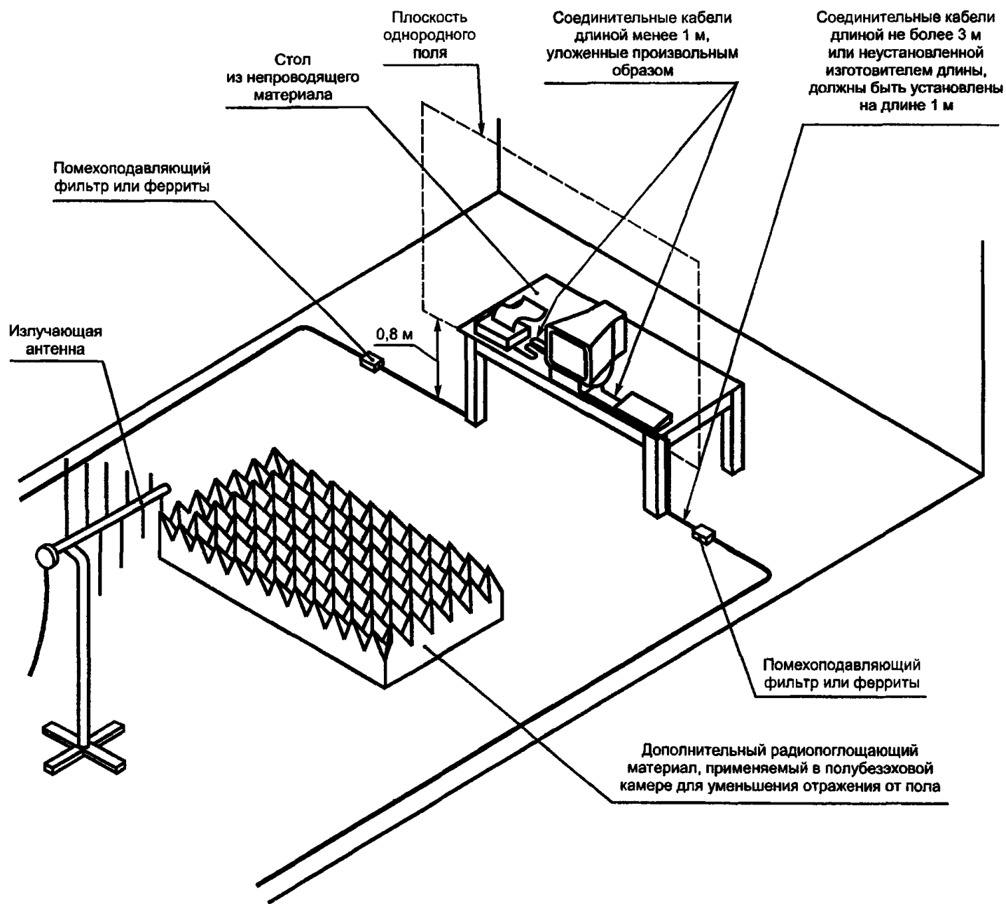
Рисунок 6 — Пример рабочего места для испытаний настольных ТС
