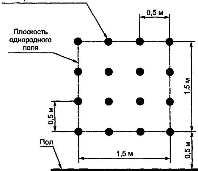
Рисунок 4 — Размеры плоскости однородного поля
