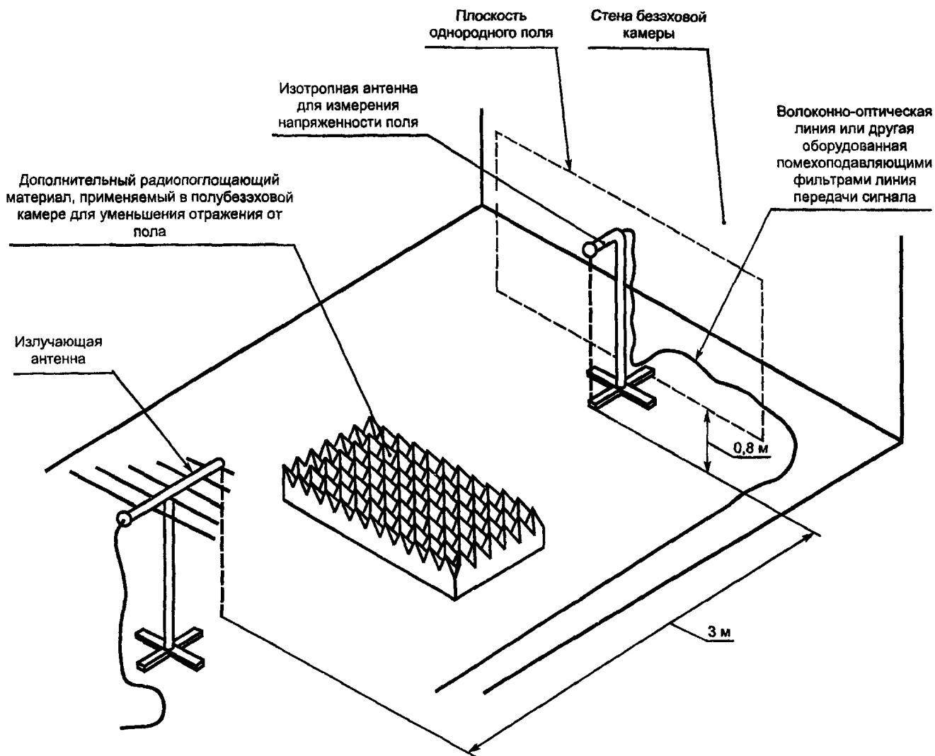
Рисунок 3 — Расположение оборудования при аттестации
