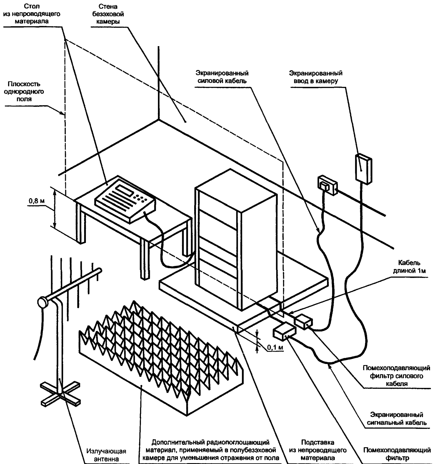
Рисунок 5 — Пример рабочего места для испытаний напольных ТС
