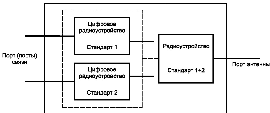
Рисунок 2 — Многокантовое радиооборудование с общим радиоинтерфейсом
