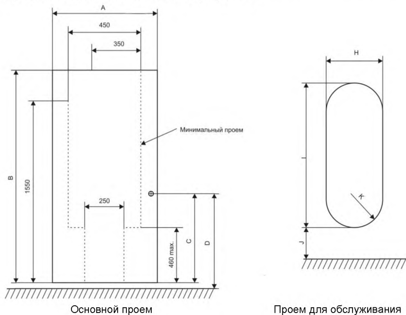
Рисунок 1 – Проемы
